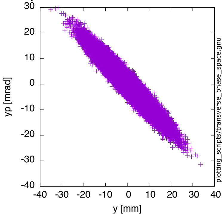
lost_muons-DistStartInjLine.dat
