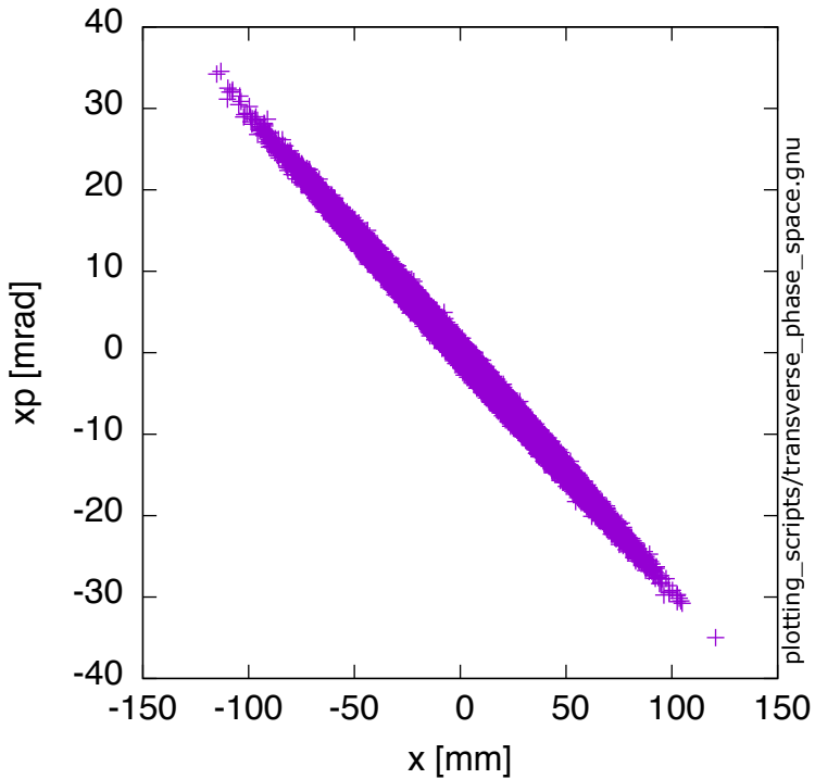
lost_muons-DistStartInjLine.dat
