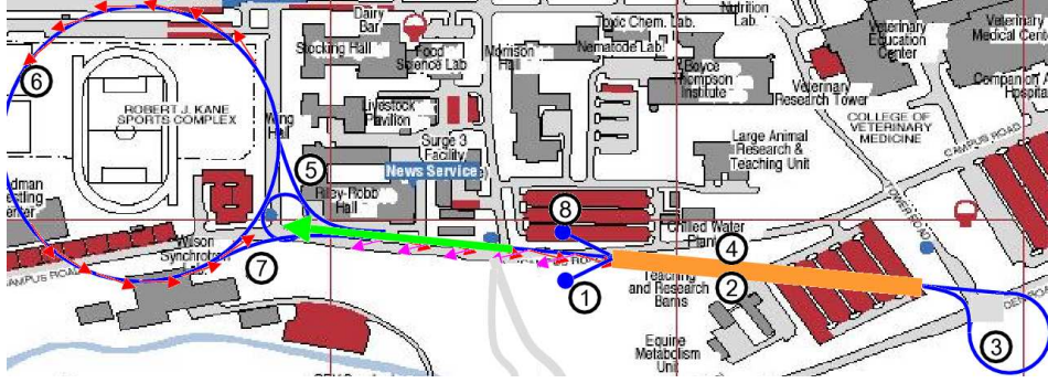
Fig. 1. An ERL in an extended CESR tunnel.
